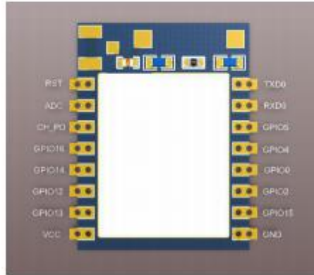
图 2 ESP-07 管脚图
