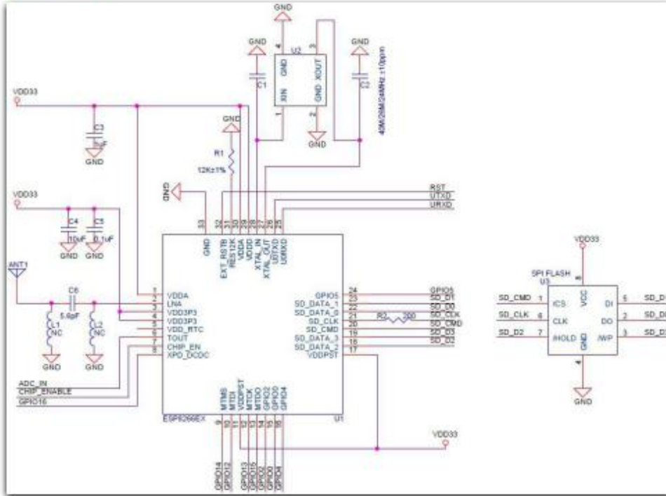
图 5 ESP-07 原理图
