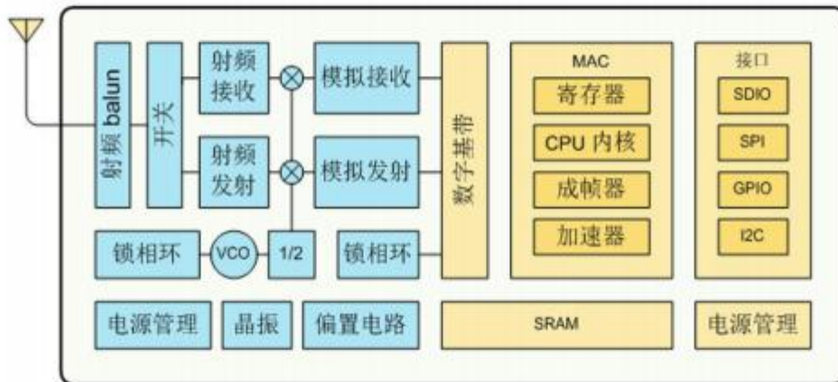
图 1 ESP8266EX 结构图
